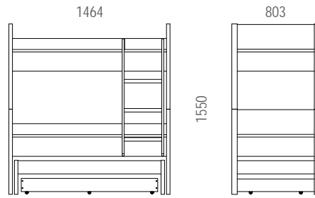
ETAGENBETT FÜR KINDER, zweiteilig
